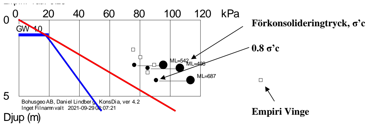
Figur 2: Konsolideringsdiagram för punkt 16.
