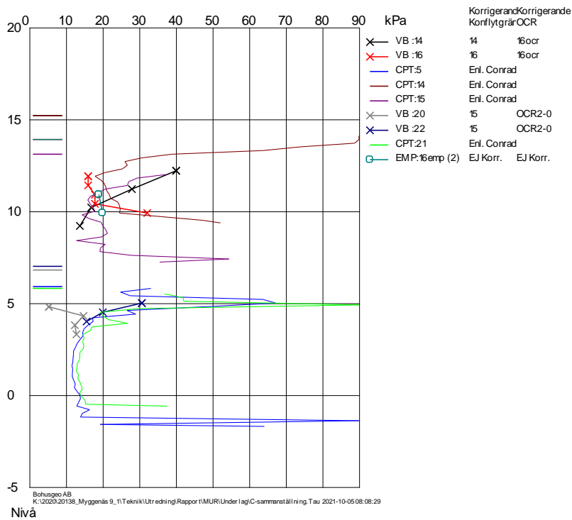
Figur 1: Sammanställning av korrigerad skjuvhållfasthet mot nivå.
